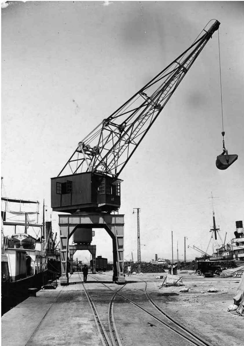
ACPT. Grua pòrtic del moll Paral·lel dotada amb calderons enlloc de les culleres automàtiques posteriors. Autor desconegut. Cap a 1933.
