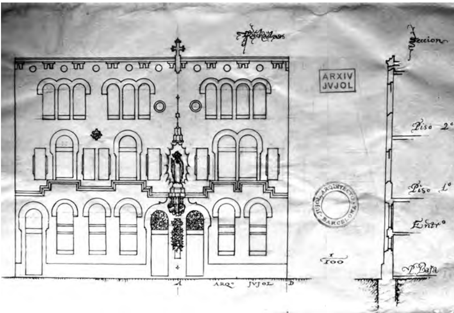
Plànol de la façana amb seccions. Arxiu Jujol.
