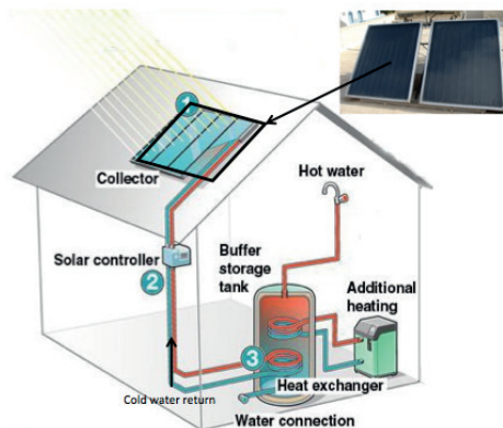
Figura 12. Absorció tèrmica solar: escalfament de l'aigua domèstica
