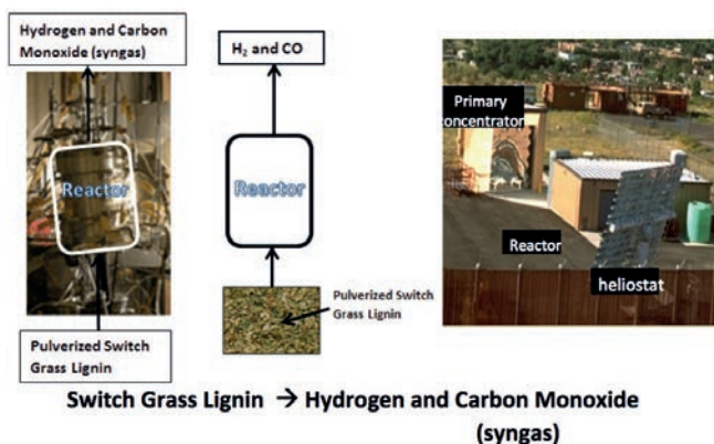
Figura 17. Reactor tèrmic solar a la Universitat de Colorado
