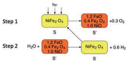
Figura 24. Fotocatàlisi: conversió d'energia solar i separació de l'aigua
