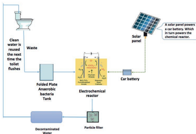
Figura 21. Lavabo solar
