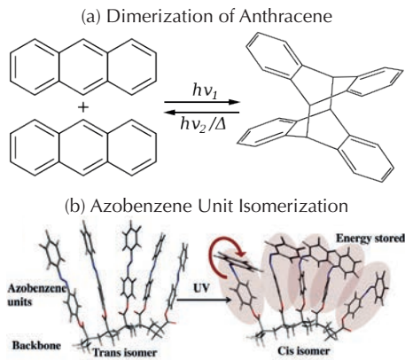
Figura 23. Química solar
